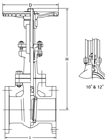
F-F dimension : JIS B 2002 End flanges : JIS B 2239 10K
